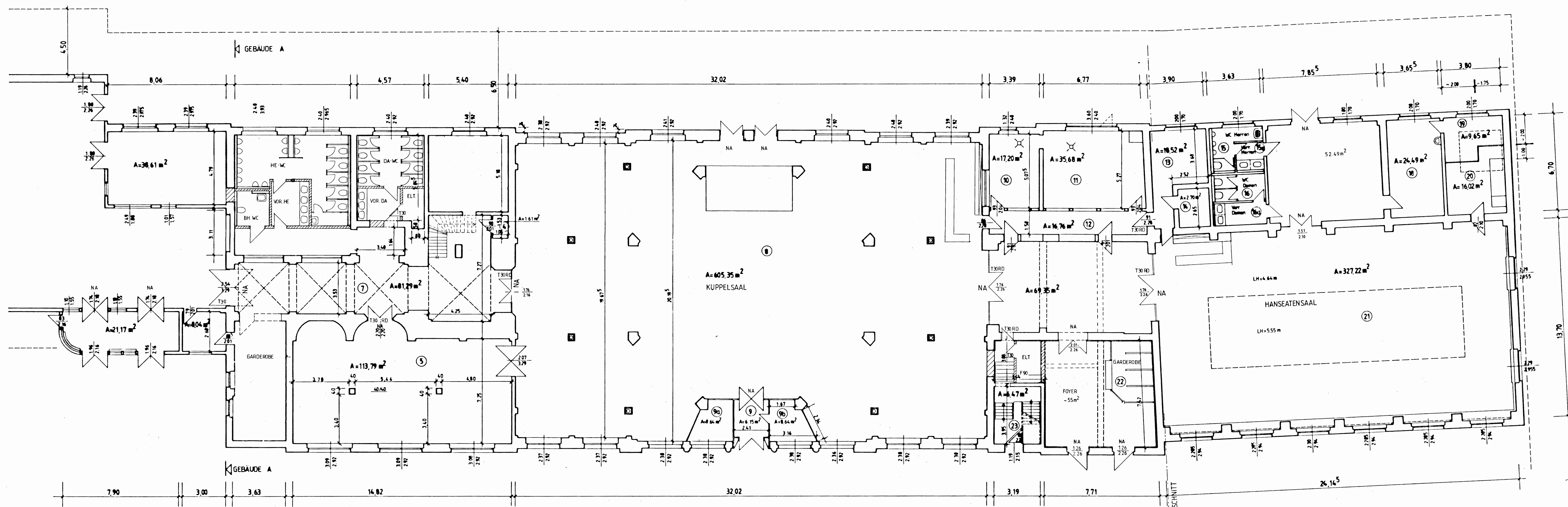
GRUNDRISS ERDGESCHOSS
